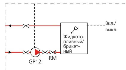
Жидкотопливный/брикетный бойлер
