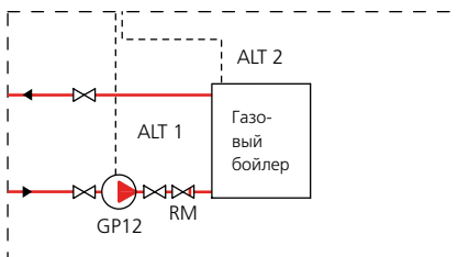
Газовый бойлер
